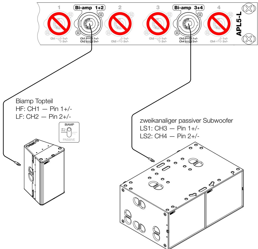
Abbildung: 4.2.1 - Biamp-Lautsprecherverkabelung
