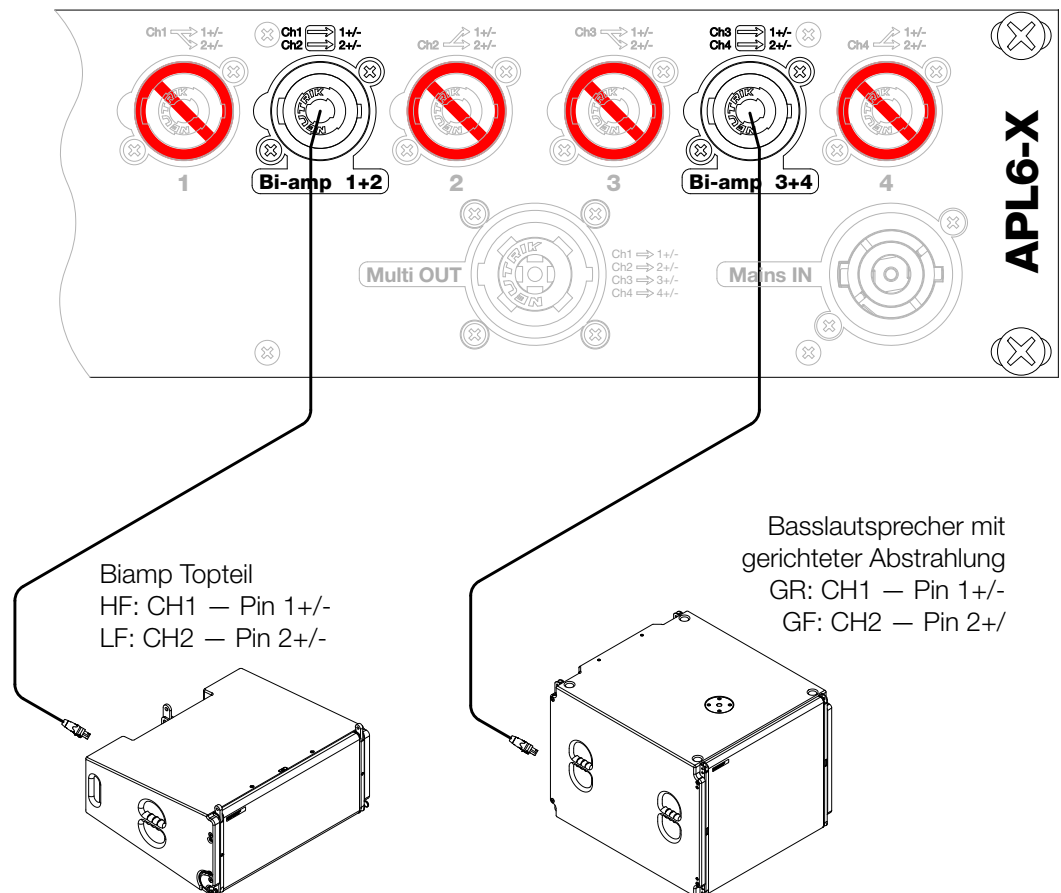
Abbildung: 4.2.2 - Biamp-Lautsprecherverkabelung
