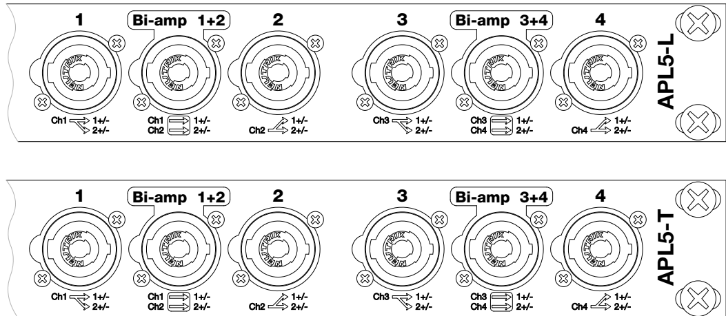
Abbildung: 2.1.3 - verkürzte Darstellung APL5-L sowie APL5-T
