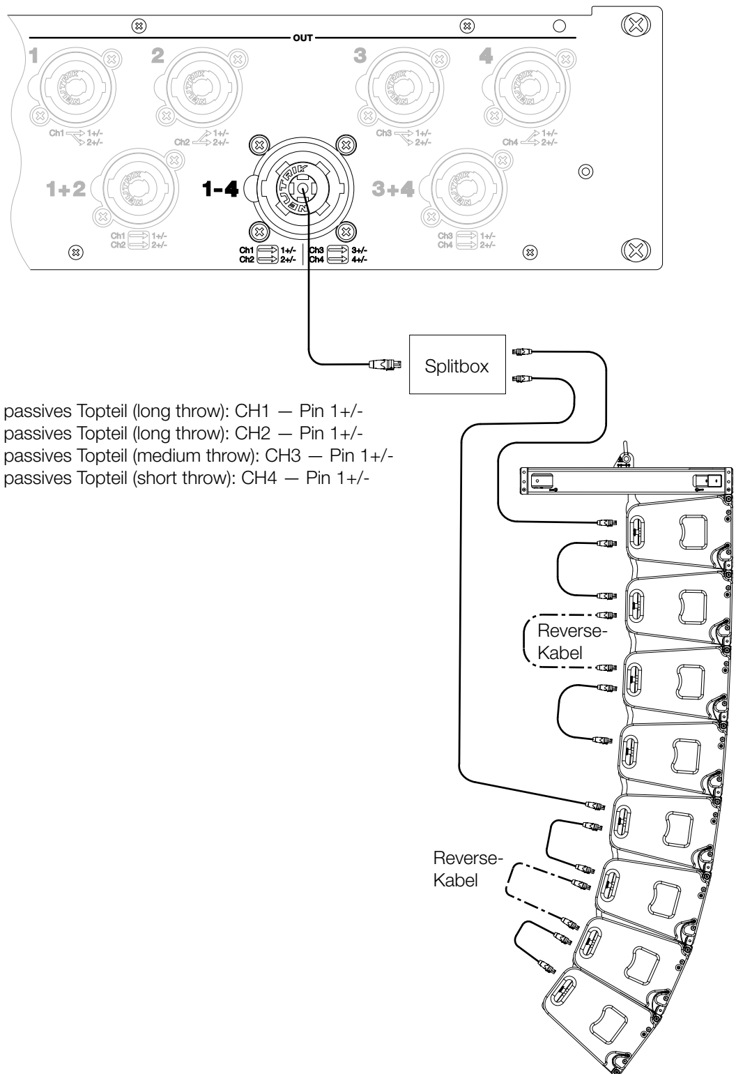
Abbildung: 4.6 - Verkabelung einkanaliges, passives Topteil mit Multi-Out
