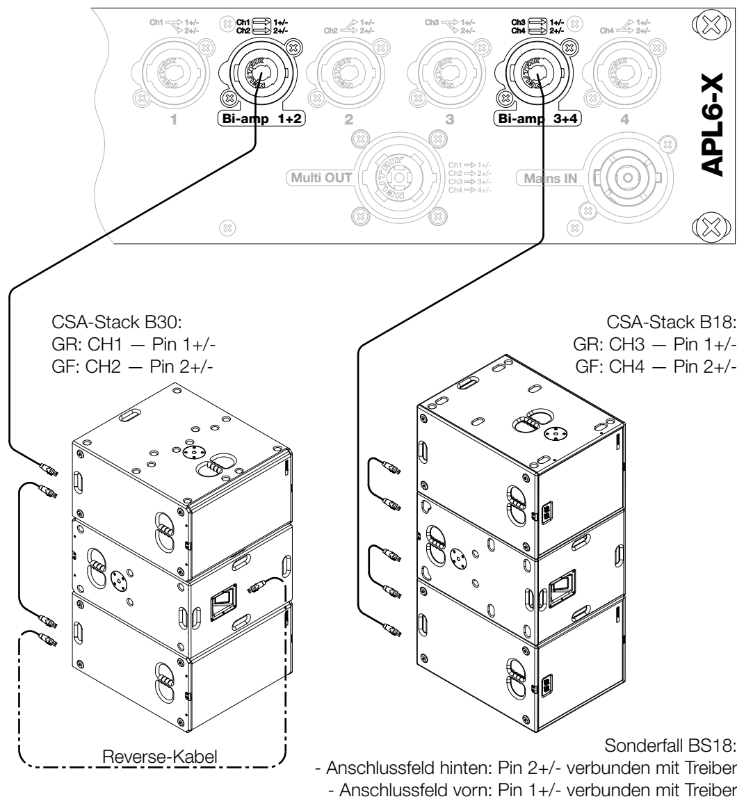
Abbildung: 4.4.1 - Verkabelung einer zweikanaligen Subwooferkonfiguration mit gerichteter Abstrahlung, Cardioid-Stack
