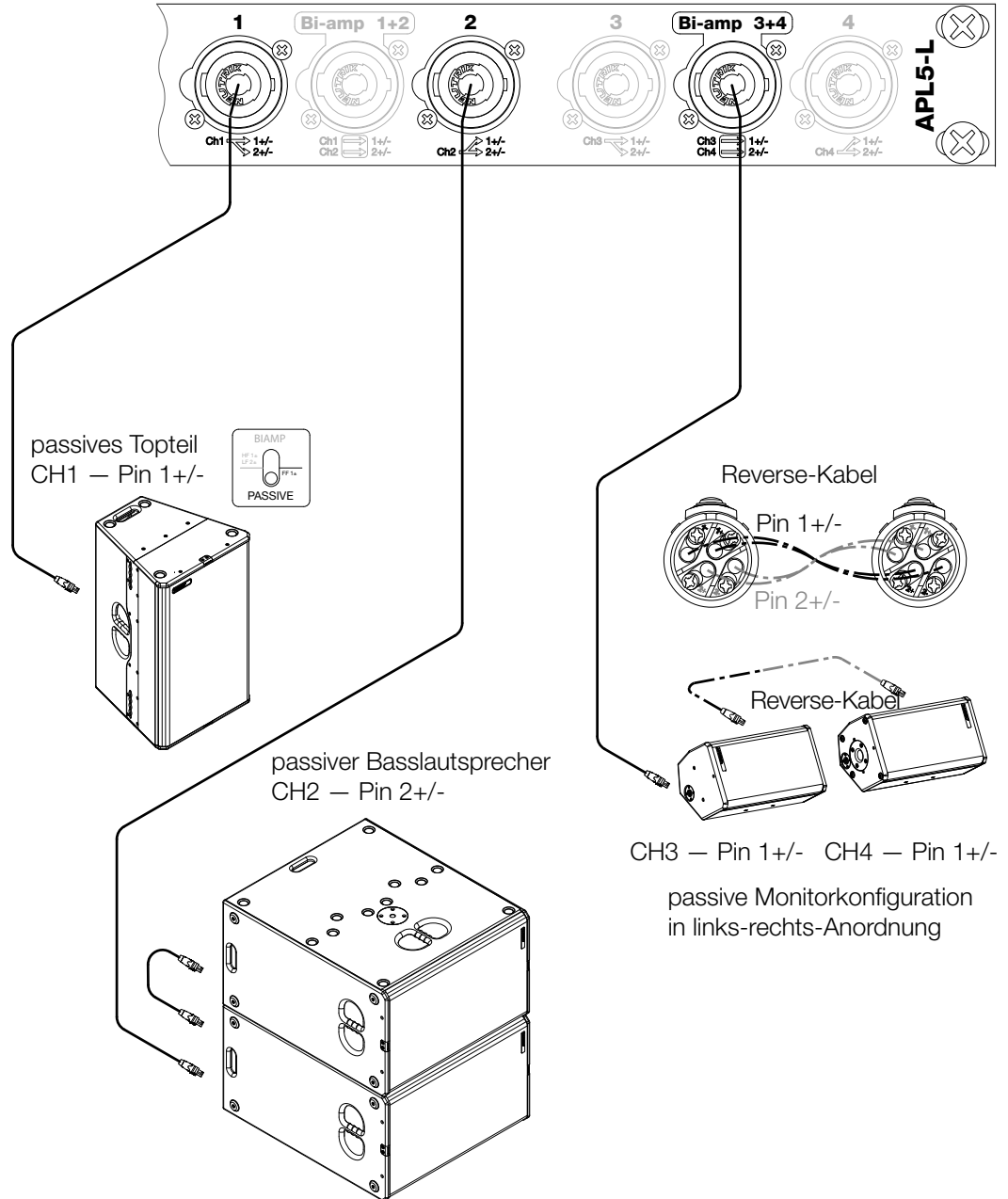
Abbildung: 4.1 - Verkabelung von einkanaligen, passiven Lautsprechern
