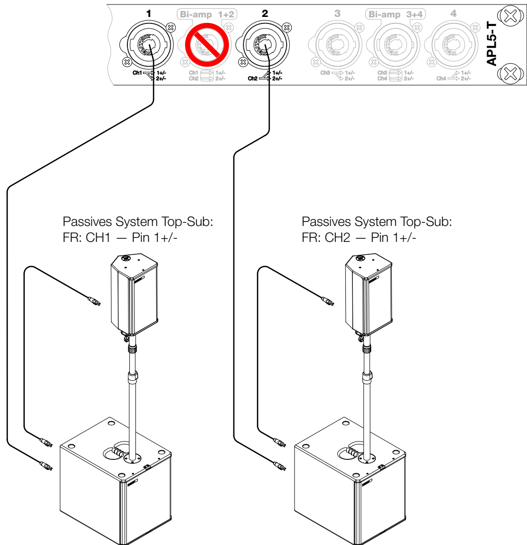
Abbildung: 4.3.2 - Verkabelung einkanaliges, passives System
