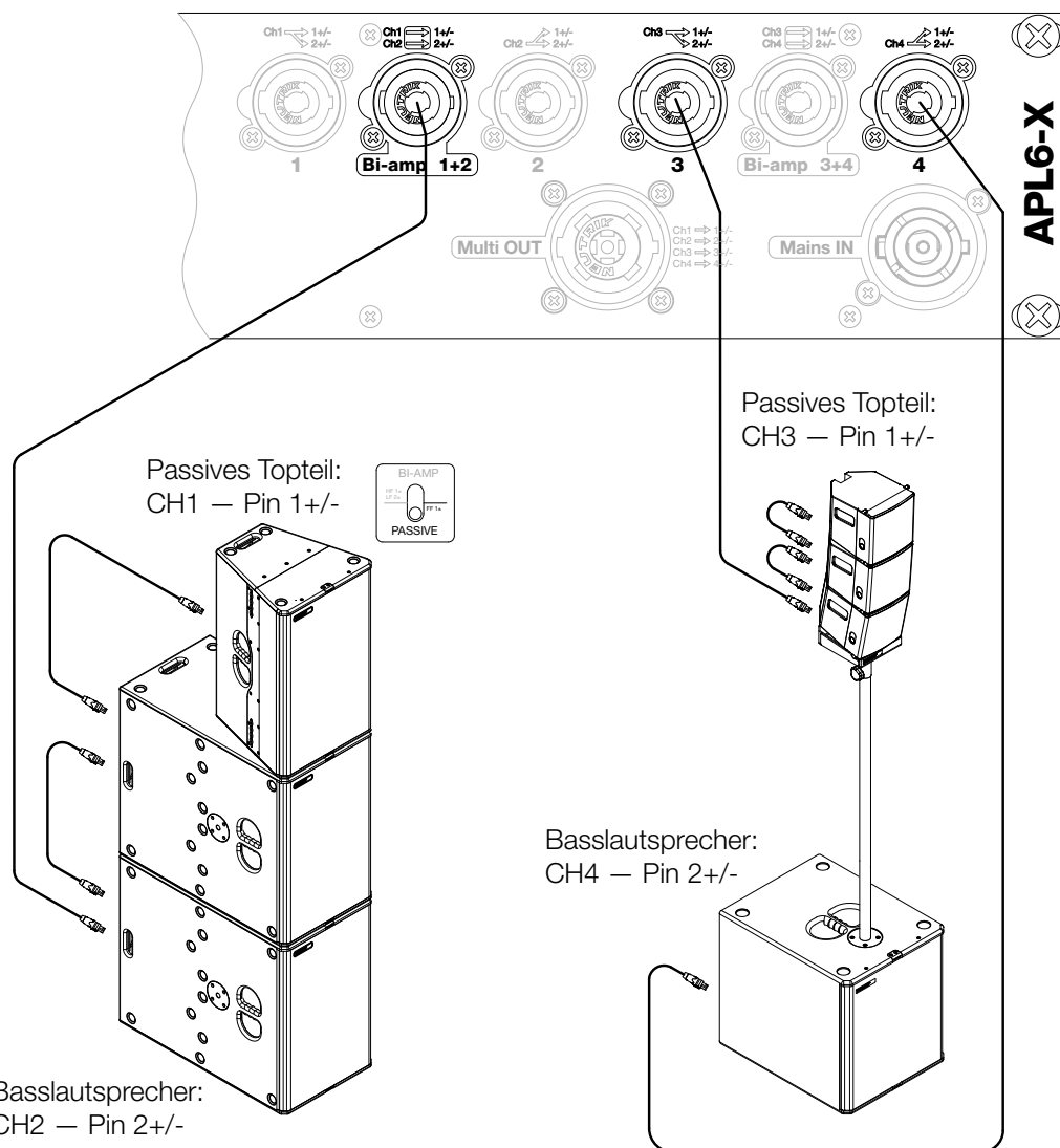
Abbildung: 4.3.1 - Verkabelung zweikanaliger, passiver Systeme
