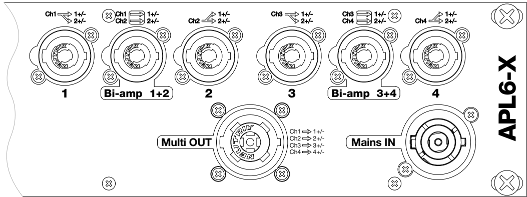
Abbildung: 2.2.2 - verkürzte Darstellung APL6-X
