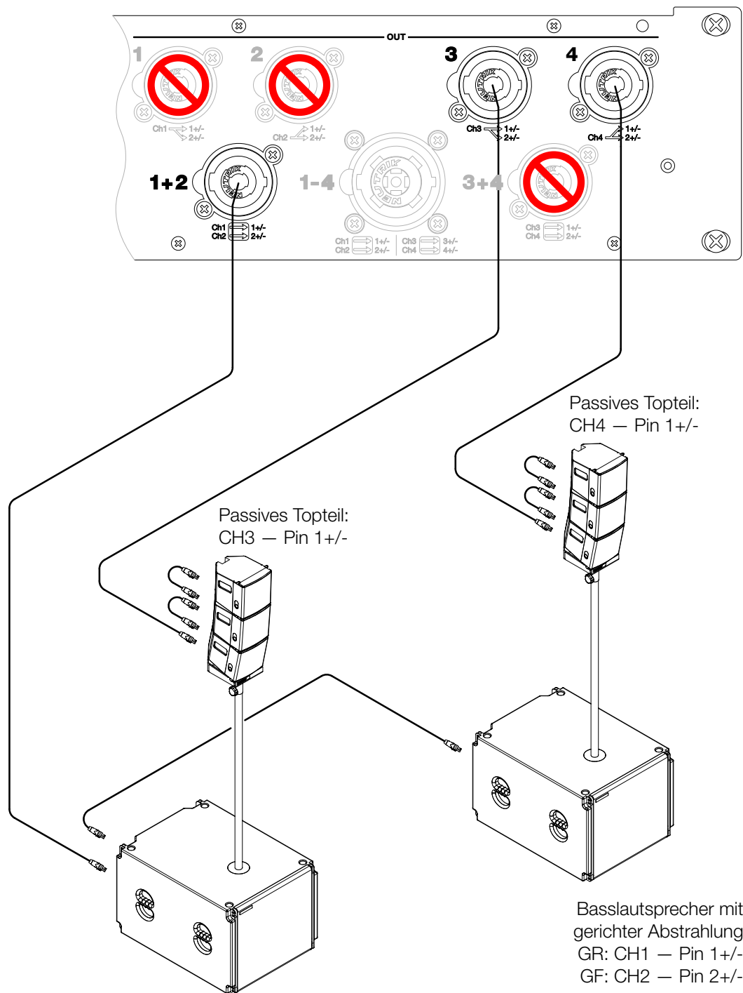
Abbildung: 4.5 - Verstärker-Systemkonfiguration mit zweikanaligem, passiven Subwoofer
