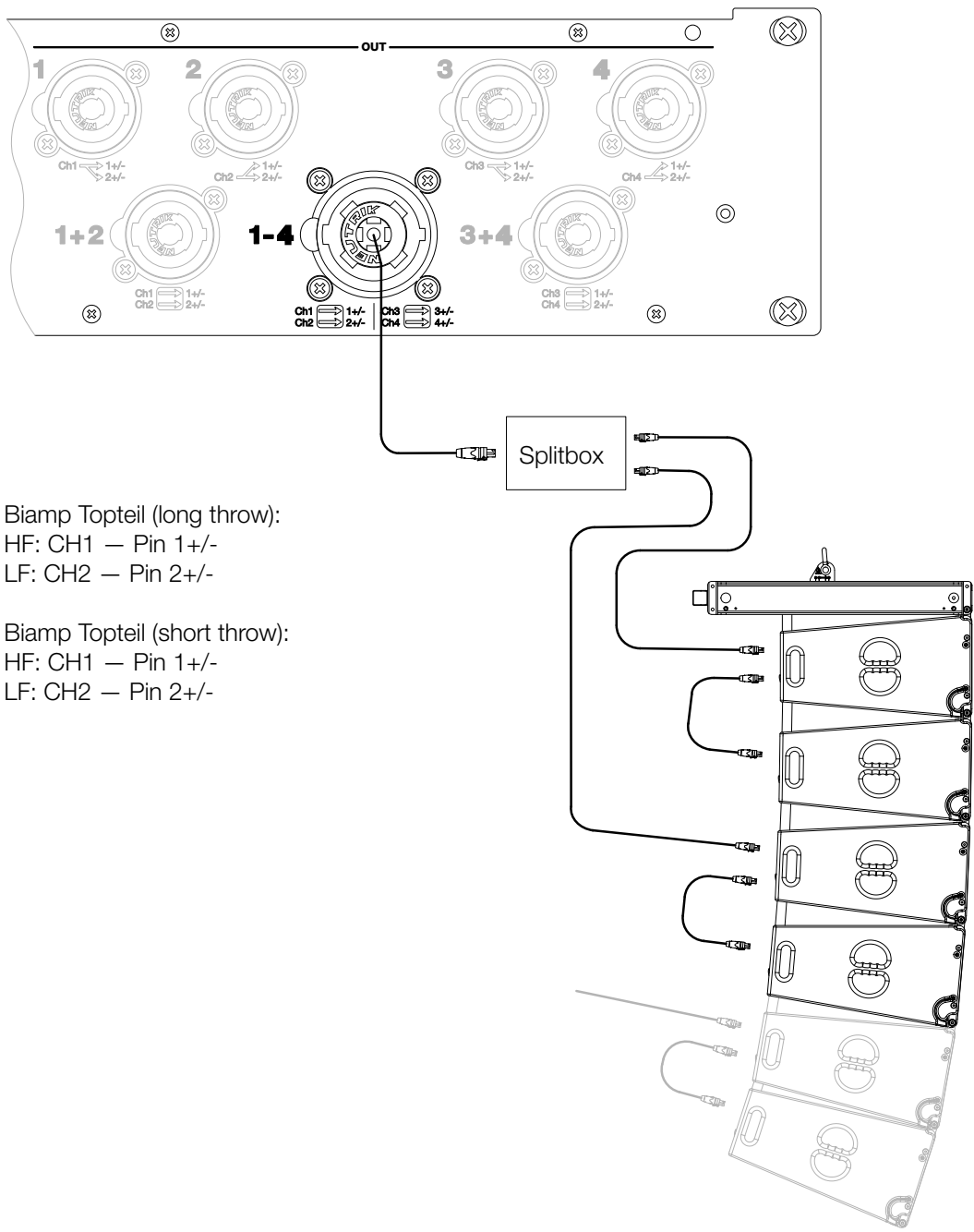
Abbildung: 4.7 - Verkabelung zweikanaliges, passives Topteil mit Multi-Out
