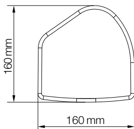
Draufsicht
