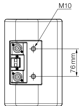
Rückansicht
