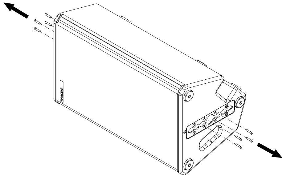
Abbildung 4.4.1 - Entfernen der Senkschrauben am M12 Lautsprecher
