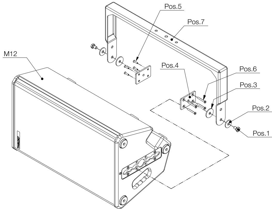
Abbildung 4.4.2 - Montage QBM12 an M12 Lautsprecher
