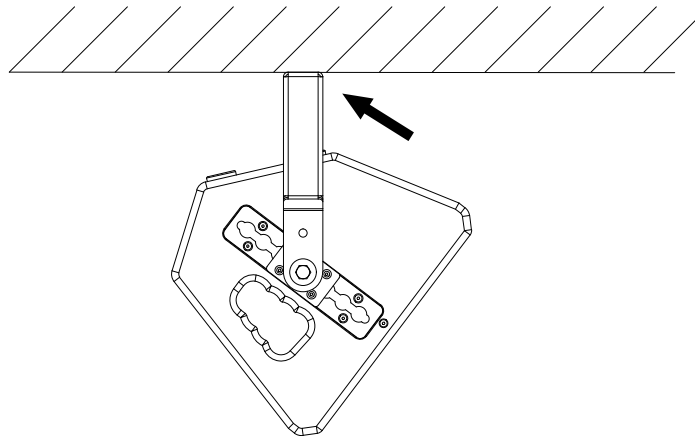
Abbildung 4.5 - QBM12 mit M12 an Decke montiert
