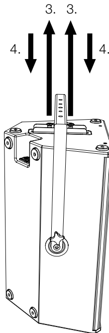
Abbildung 4.3 - Montage SBM15 an M15 Lautsprecher
